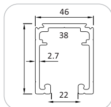
Top Track : CASP-T1
