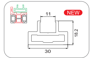
CASP-SP-3010 - DOOR FRAME PROFILE
