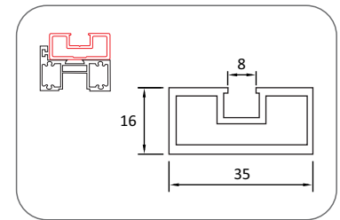
CASP-SP-3516 - DOOR FRAMED PROFILE
