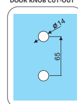
DOOR KNOB CUT-OUT
