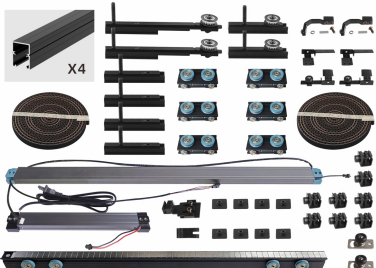
CASP-MT09 - 1 Fix+3 Slide Max Door Width : 1150 mm ₹: 235000/-*
