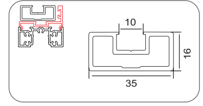
CASP-SP-3516 - DOOR FRAMED PROFILE
