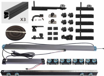
CASP-MT08 - 1 Fix+2 Slide Max Door Width : 1150 mm ₹: 215000/-*
